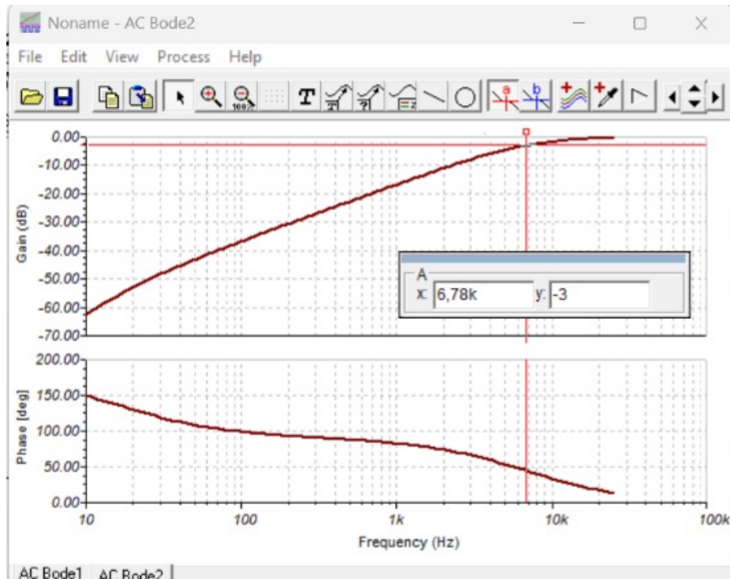
Figura 27: Simulación del HPF fcut max.
