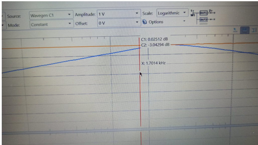
Figura 17: Bode del filtro High.
