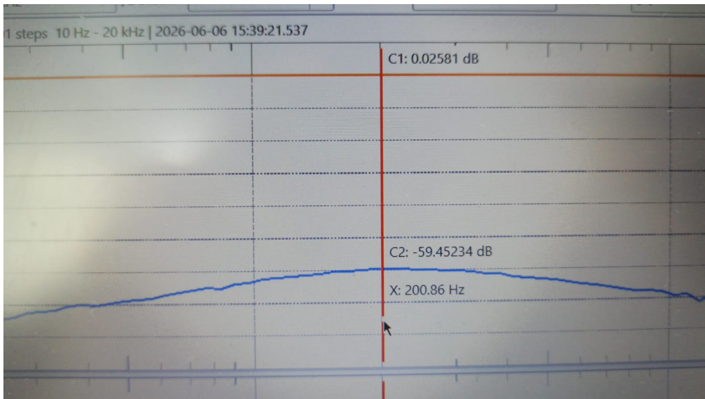
Figura 8: Diagrama 2 de Bode del filtro Bass.
